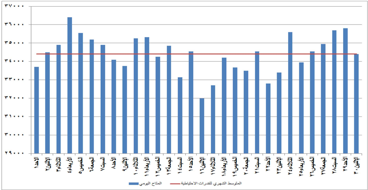
شكل (٢٧) القدرات المتاحة يوميا والمتوسط الشهري للقدرة الاحتياطية خلال شهر ابريل ٢٠١٨
