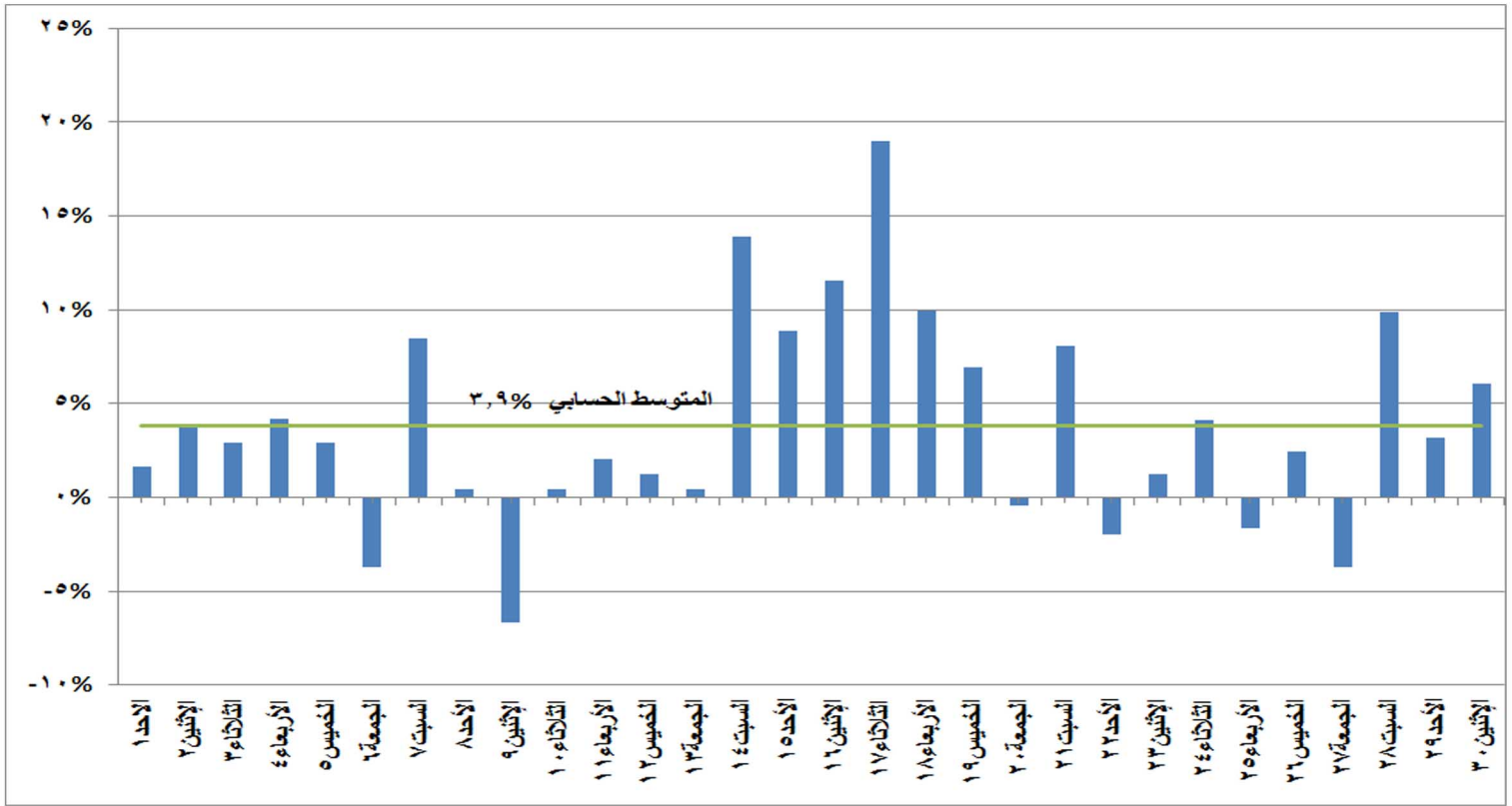
شكل (٩) النسب المئوية للتغير في الحمل الاقصى خلال شهر ابريل ٢٠١٨ مقارنة باليوم المماثل من العام الماضي
