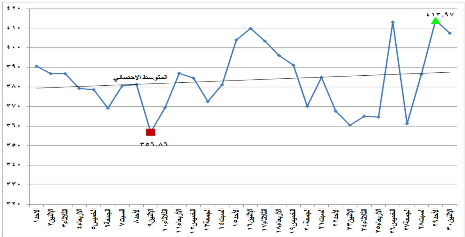
شكل (١٧) الطاقة الكهربائية المنتجة من الغاز الطبيعي خلال شهر أبريل ٢٠١٨
