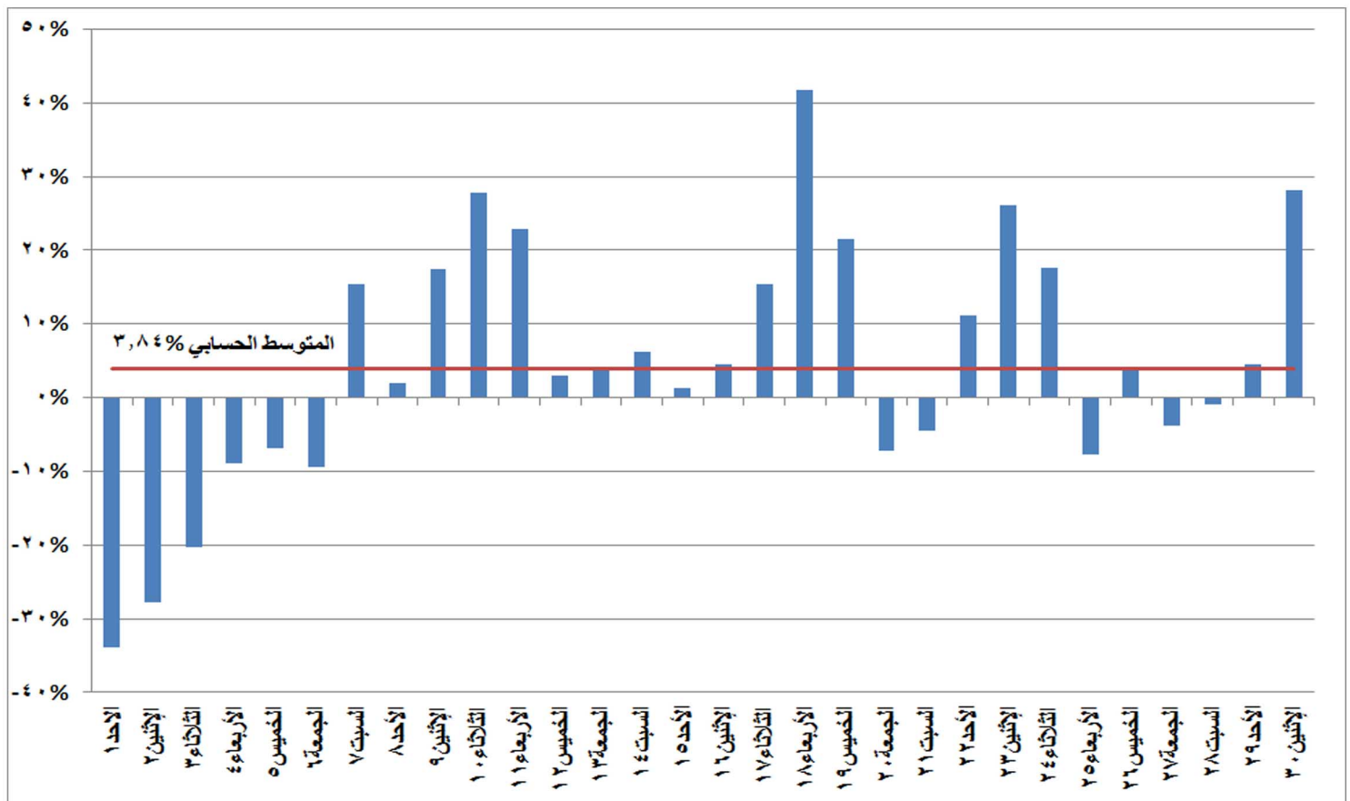
شكل (٢٠) نسب التغير في استخدام المازوت في إنتاج الطاقة الكهربائية خلال شهر ابريل ٢٠١٨ مقارنة بالشهر المماثل من العام السابق
