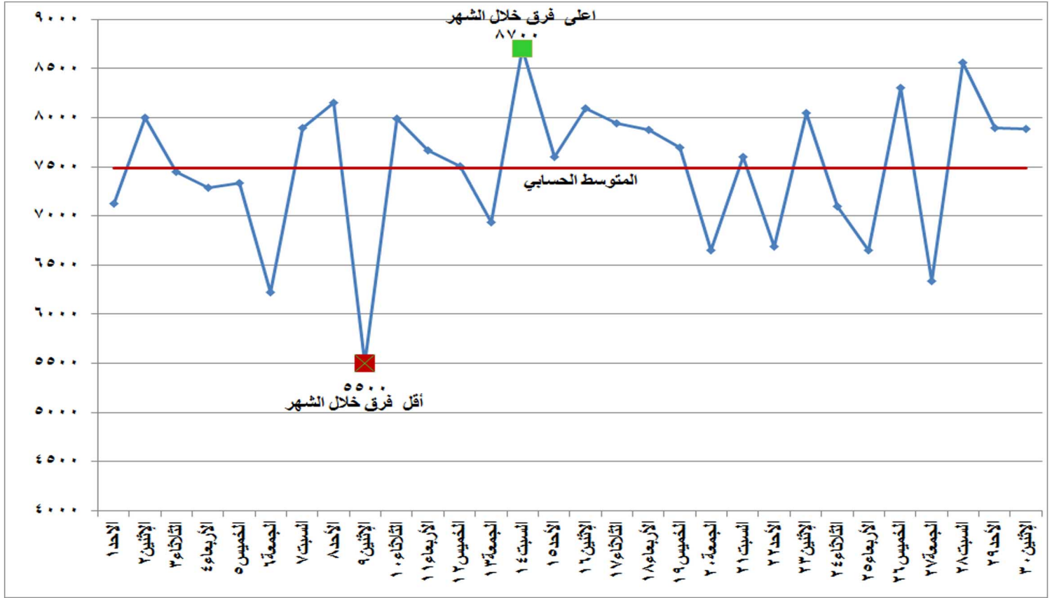
شكل (٣) الفرق بين أقصى وأدنى حمل خلال شهر ابريل ٢٠١٨
