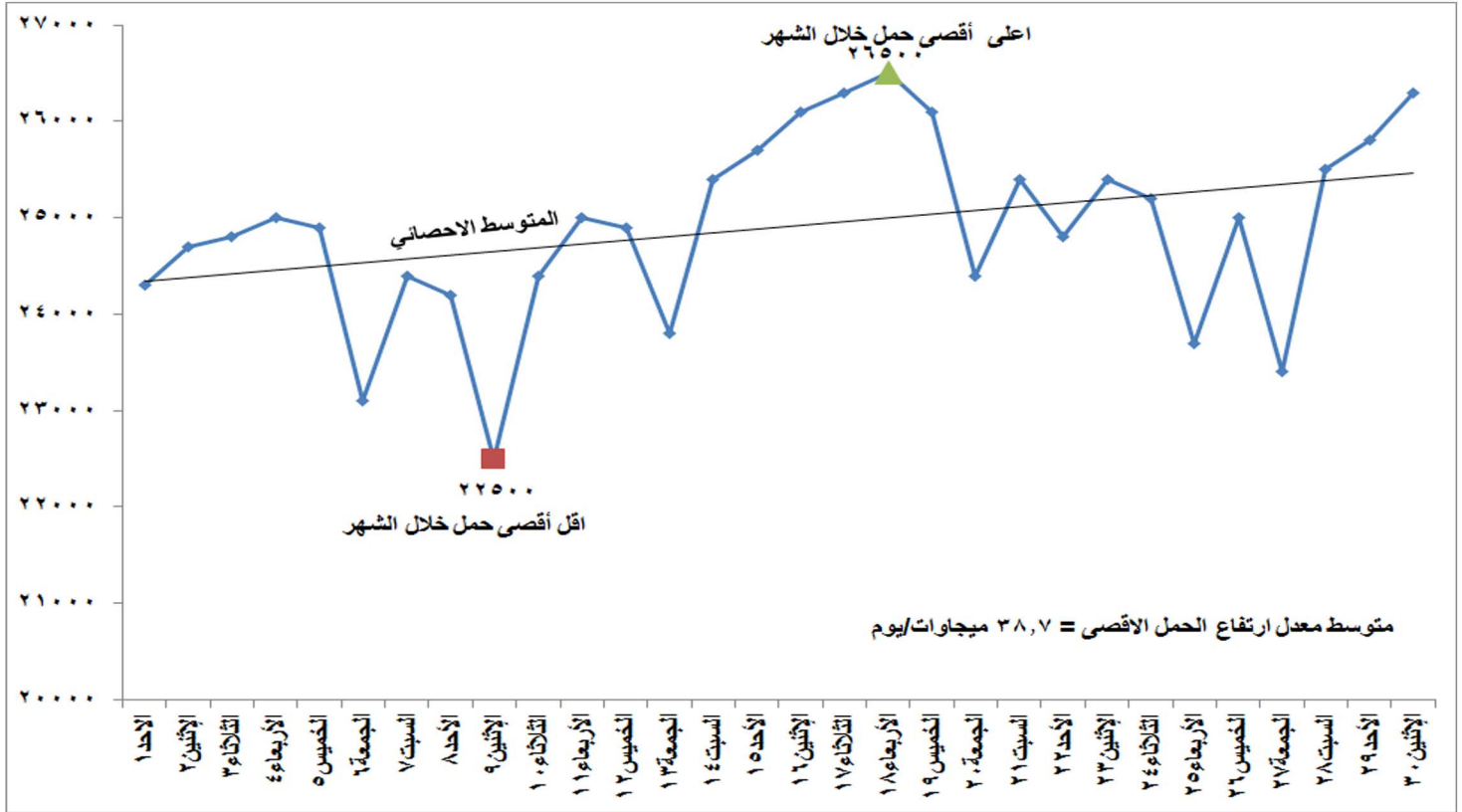
شكل (١) تطور الحمل الاقصى اليومي خلال شهر ابريل ٢٠١٨
