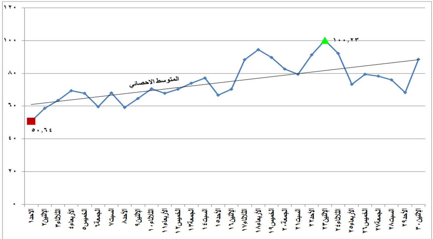
شكل (١٩) الطاقة الكهربائية المنتجة من المازوت خلال شهر ابريل ٢٠١٨
