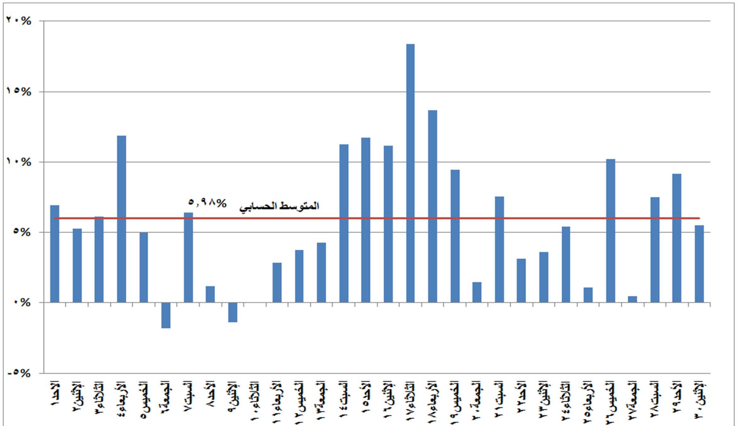
شكل (١٦) نسب التغير في الطاقة الكهربائية المنتجة خلال شهر ابريل ٢٠١٨ مقارنة بالشهر المماثل من العام السابق
