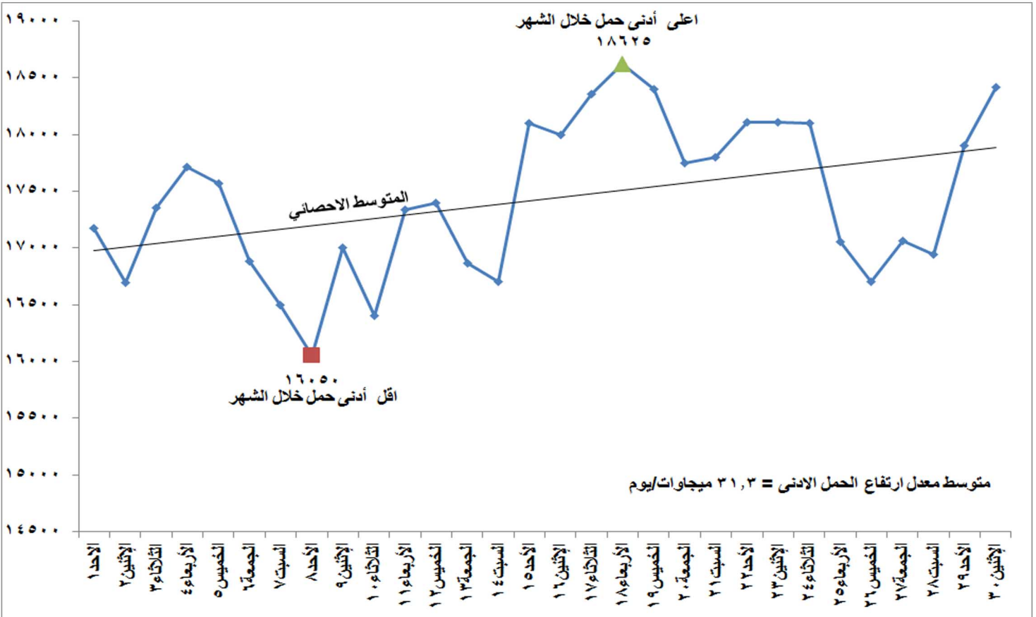
شكل (٢) تطور الحمل الادنى اليومي خلال شهر ابريل ٢٠١٨
