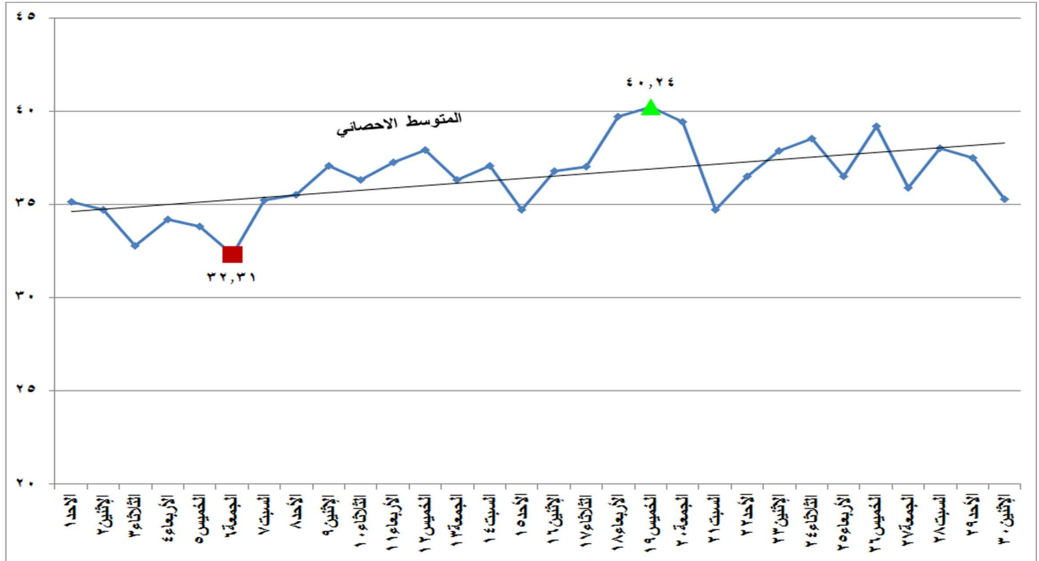
شكل (٢٣) الطاقة الكهربائية المنتجة من المصادر المائية خلال شهر ابريل ٢٠١٨
