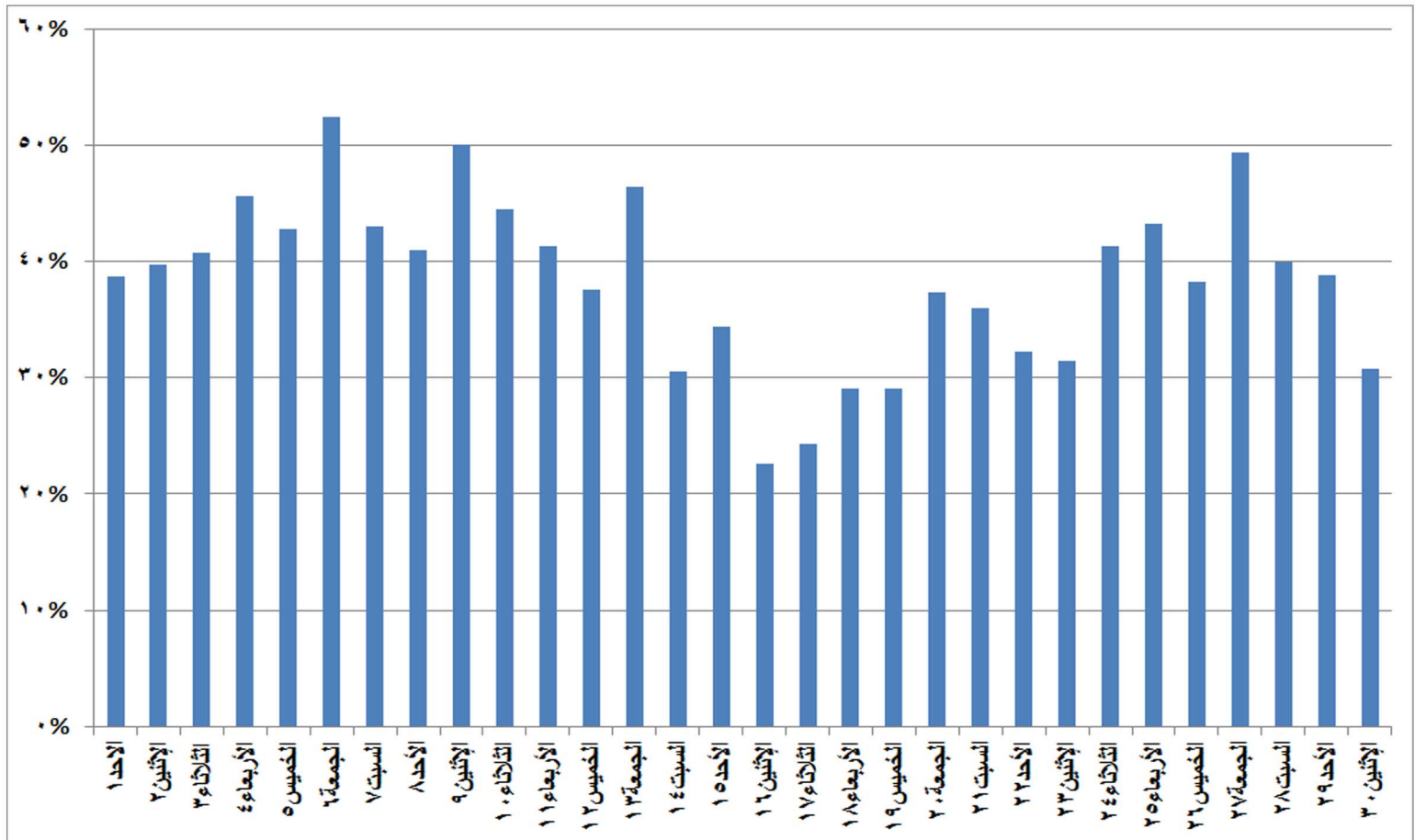
شكل (٢٨) نسب الفائض للحمل الاقصى المسجل يوميا خلال شهر ابريل ٢٠١٨
