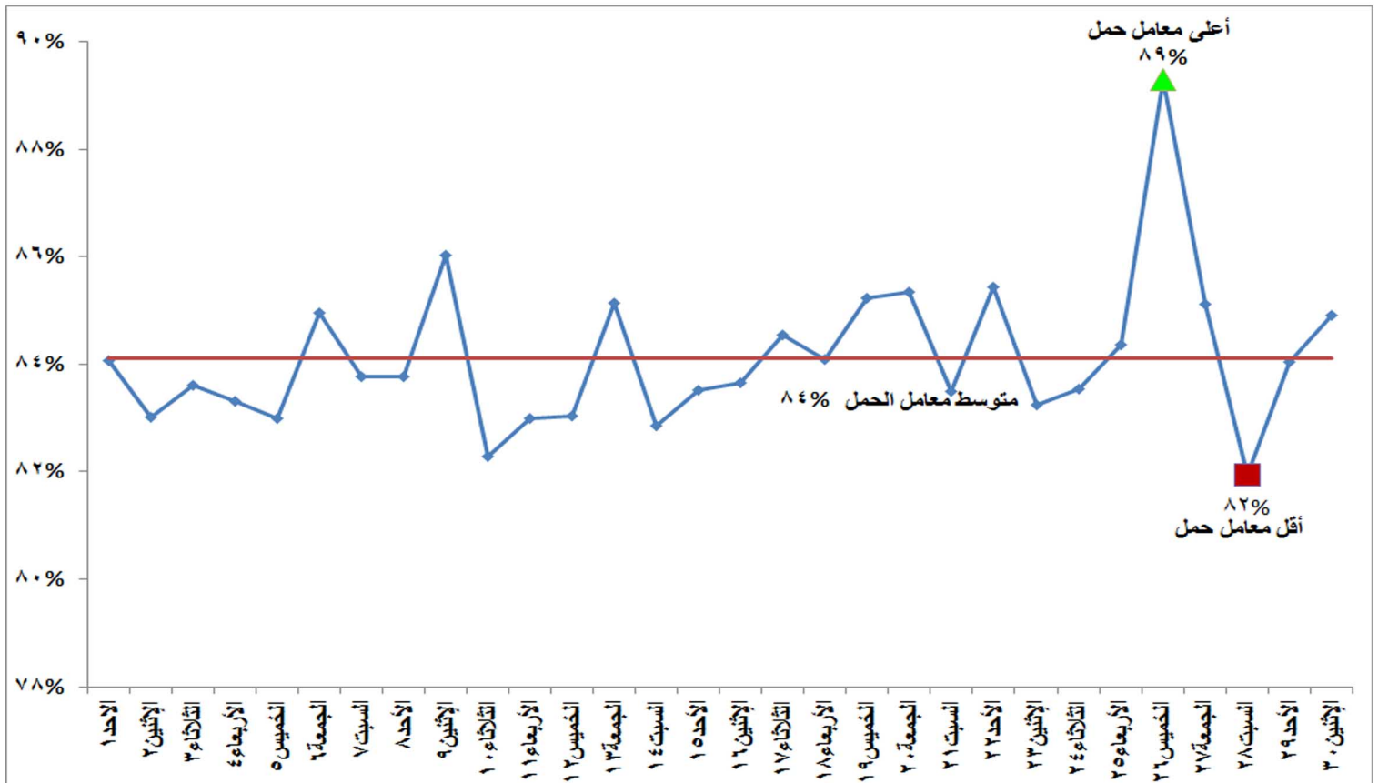
شكل (١٢) إجمالي معامل الحمل لوحدات الانتاج خلال شهر ابريل ٢٠١٨
