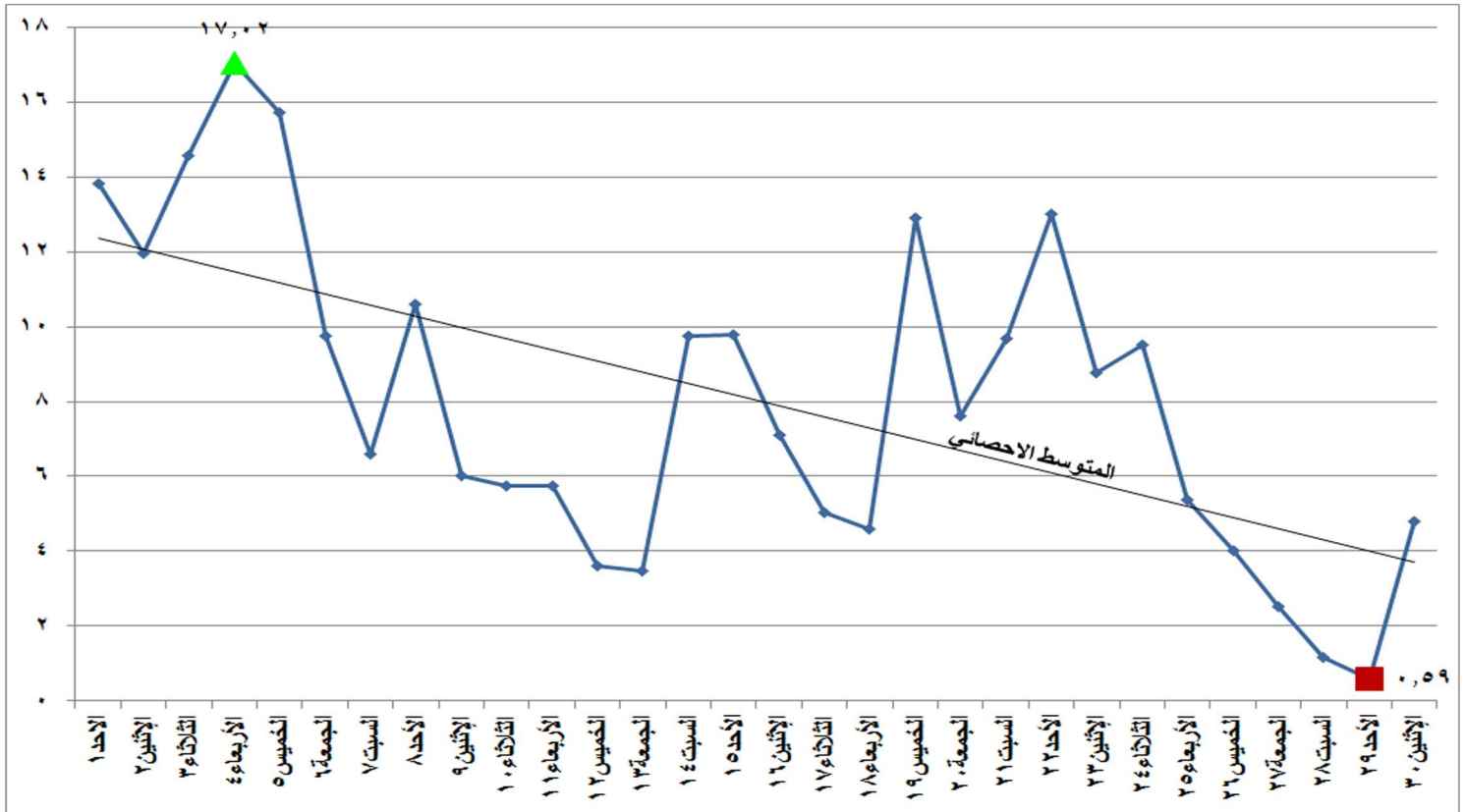
شكل (٢٥) الطاقة الكهربائية المنتجة من الرياح والشمس خلال شهر ابريل ٢٠١٨
